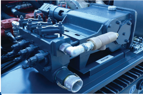
BULLDRILL güçlü çamur pompası; Dakikada 140 lt su basma kapasitesi (maks. 70 bar)
